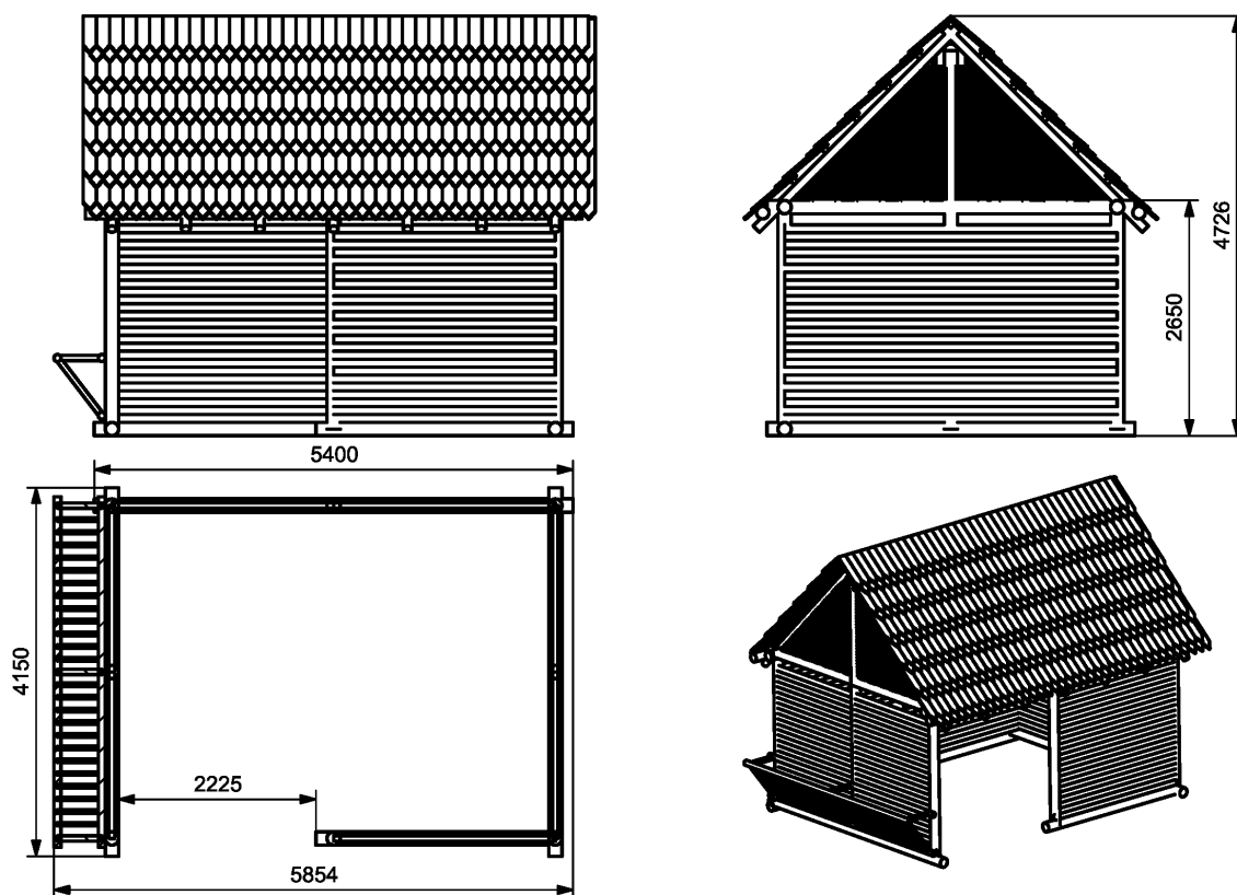
Rozměry přístřešku
