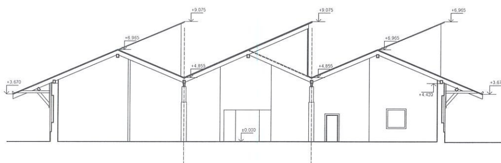
VÝŠKA INTERIERU
