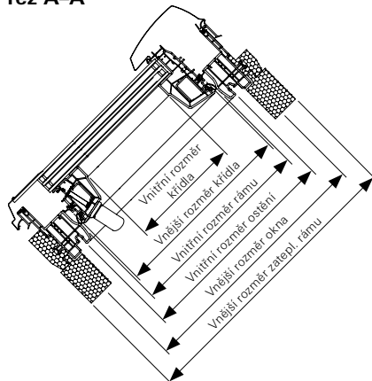
řez A–A
