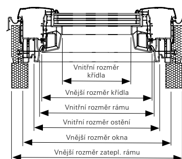
řez B–B
