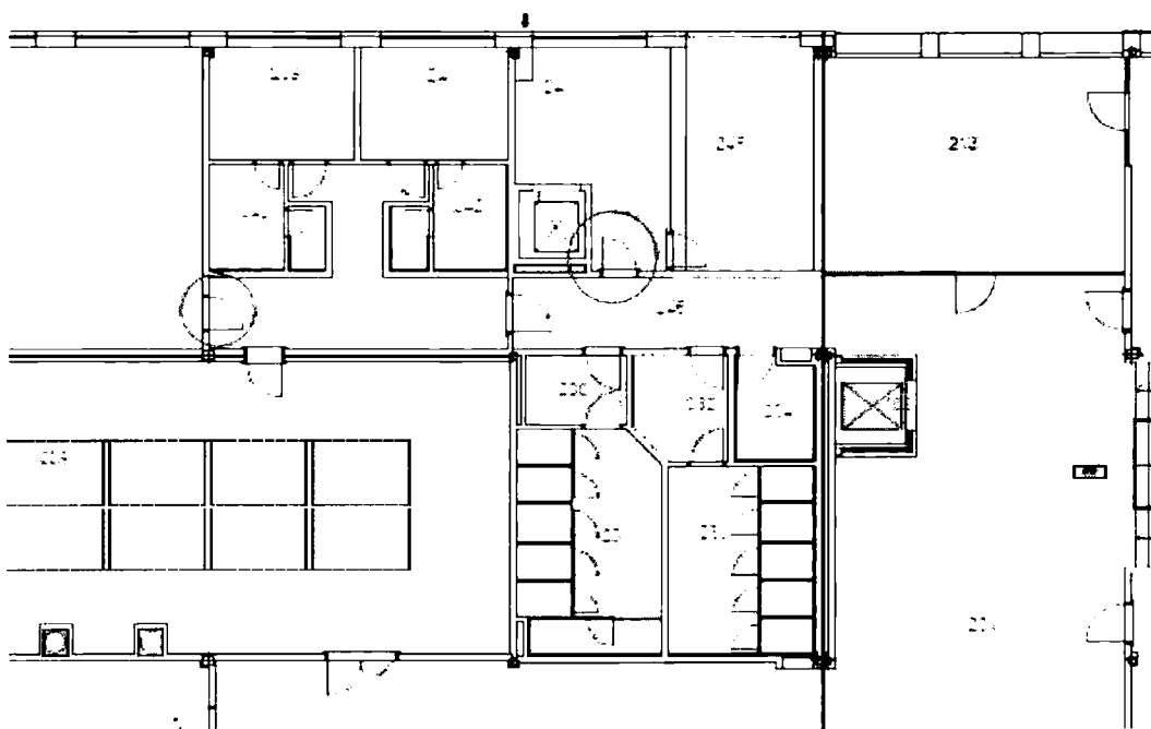
PŮDORYS 2.NP
