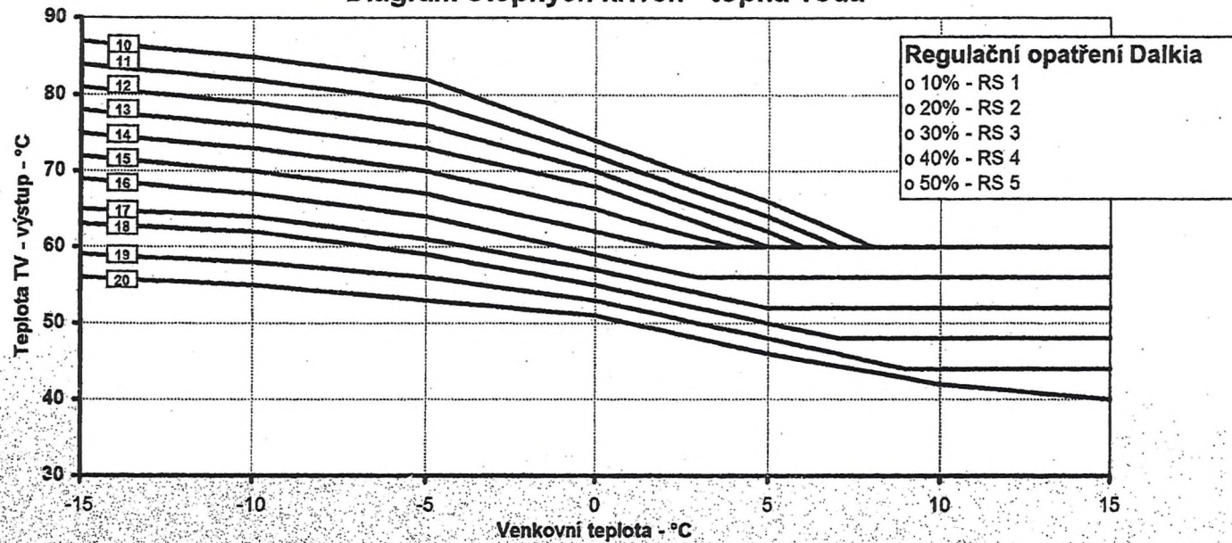
Diagram otopných křivek - topná voda
