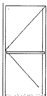
vodorovné nerez madlo 40/28, 700mm od Č.P. (pouze zevnitř)
