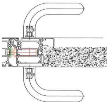
madlo typ E (380/155mm), nerez – oboustranně
