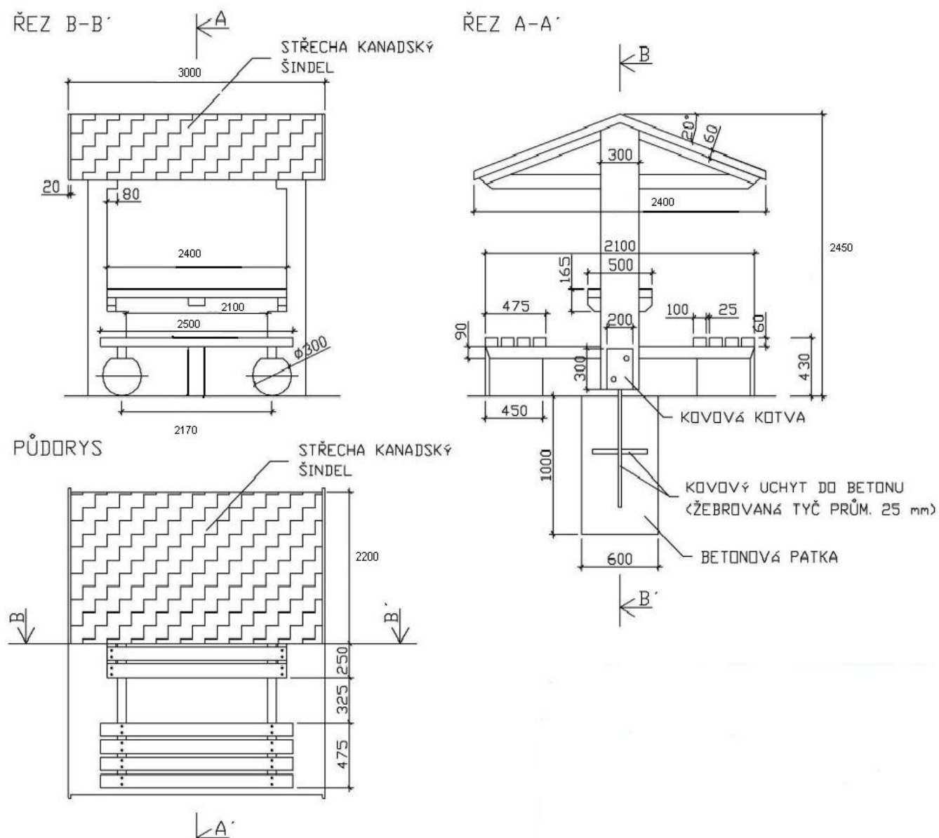
Obrázek 1: Výkres odpočinkového zařízení (altánu)
