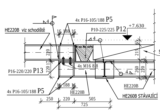
DETAIL "E" 1:25 řez
