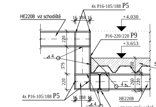
DETAIL "E" 1:25 řez
