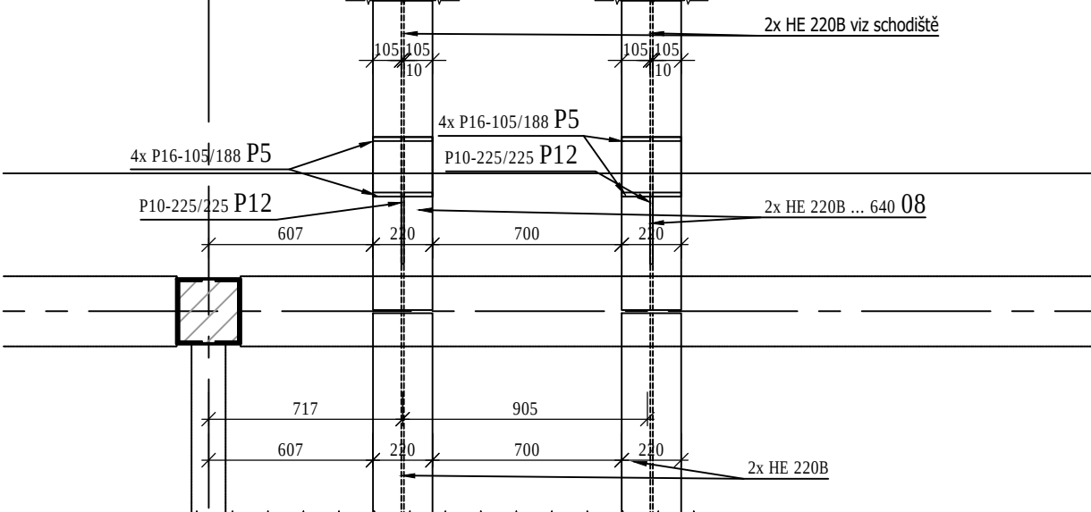
DETAIL "E" 1:25 půdorys
