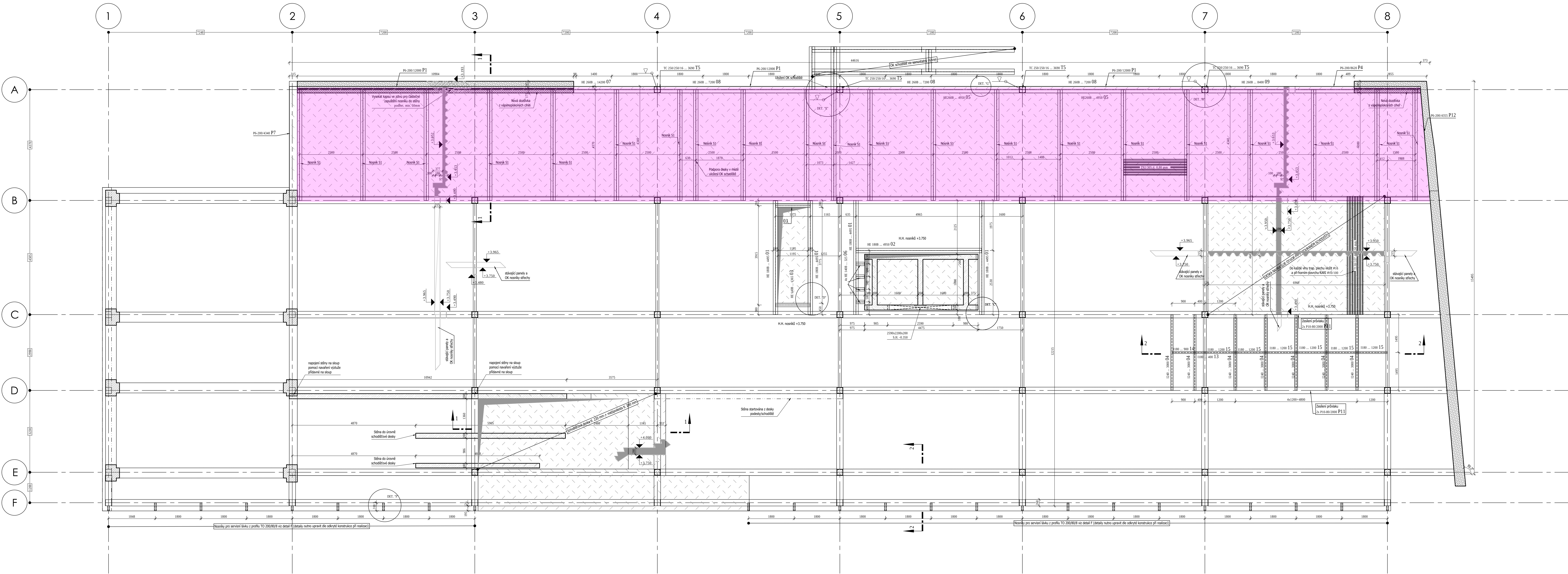
DETAIL "E" 1:25 půdorys
