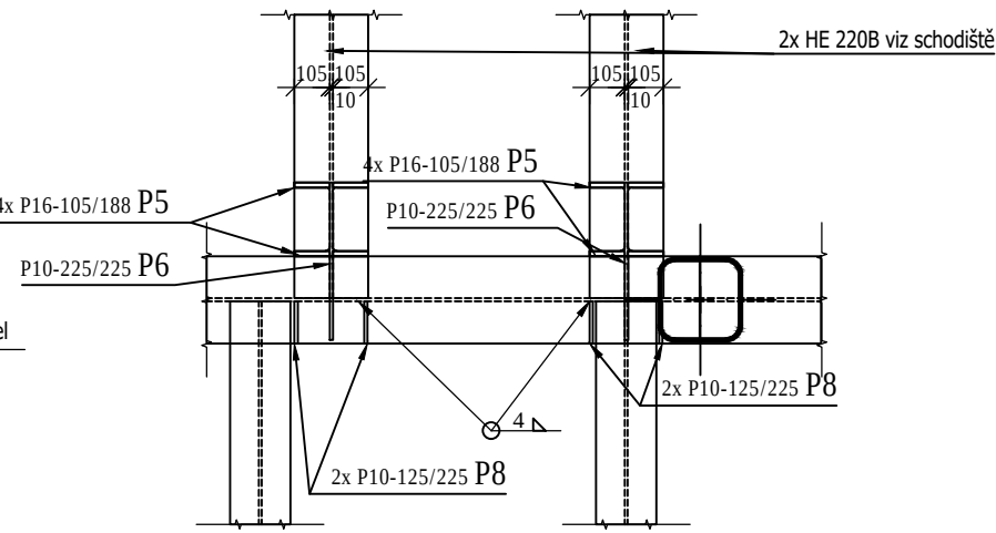
DETAIL "E" 1:25 půdorys
