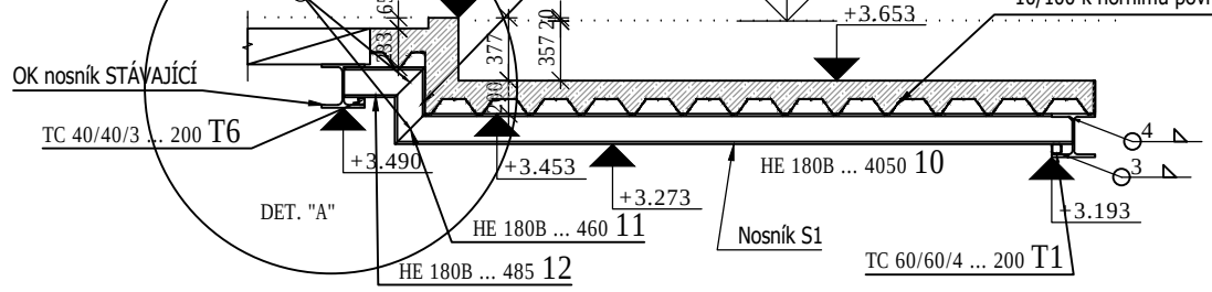
ŘEZ 1-1 NOSNÍK S1 NOVÉHO STROPU
