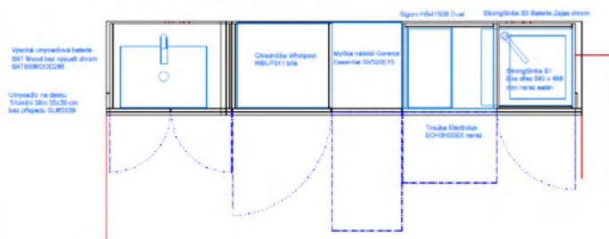
PŮDORYS SPODNÍCH SKŘÍŇEK S PLÁTEM A DŘEZEM
