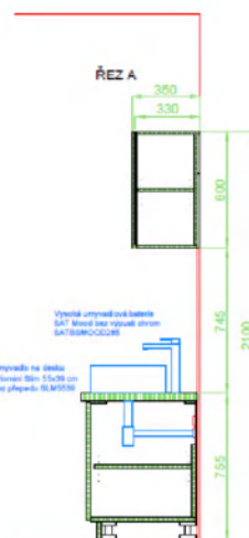
KOMODA MEZI OKNA
