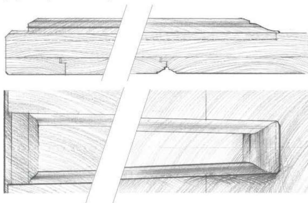
kónický rybinový svlak, stahující základní konstrukční desku dveří
