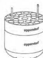
Adapter 2,6 - 8 ml
