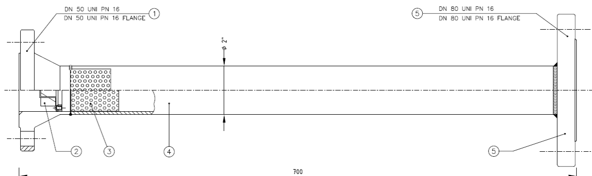
Generátor nízkoexpanzní pěny L4st, průtok 400 l/min, při tlaku 5 bar, poměr napěnění 1:7
