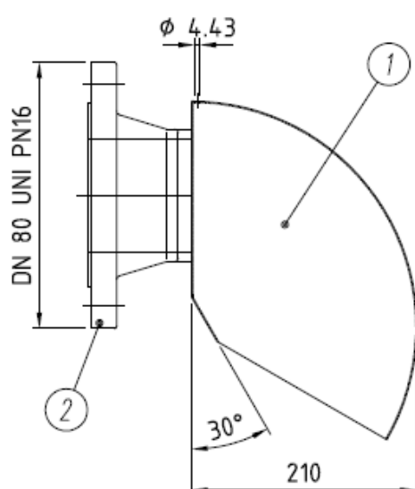
Nalévač pěny SK 80
