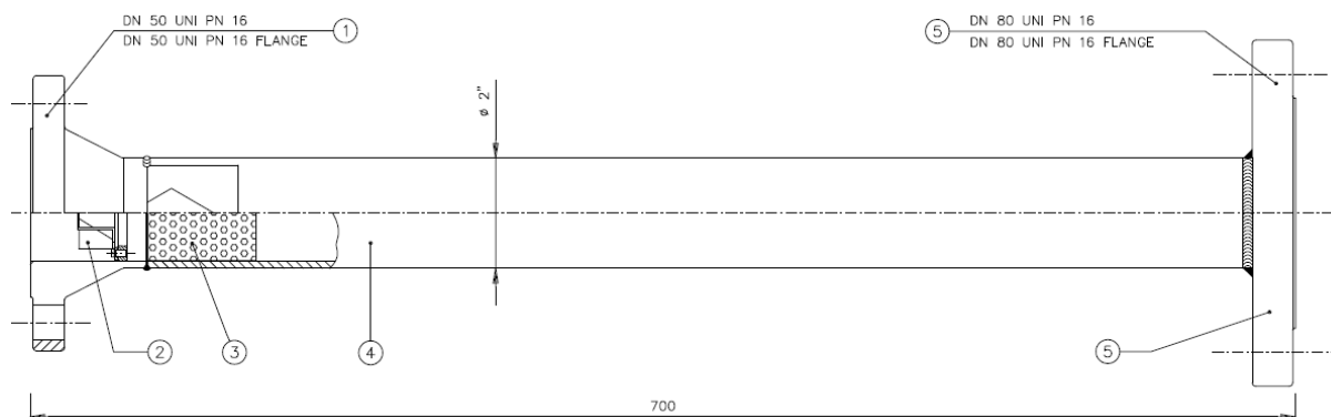
Generátor nízkoexpanzní pěny L4st, průtok 400 l/min, při tlaku 5 bar, poměr napěnění 1:7
