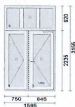
Pozice 12 Kování klíka-klíka, zámek jednobodový, RAL 9016 matná, 93 Kg. Průchozí rozměry: šířka = 759 mm, výška = 2180 mm. Zevnitř
