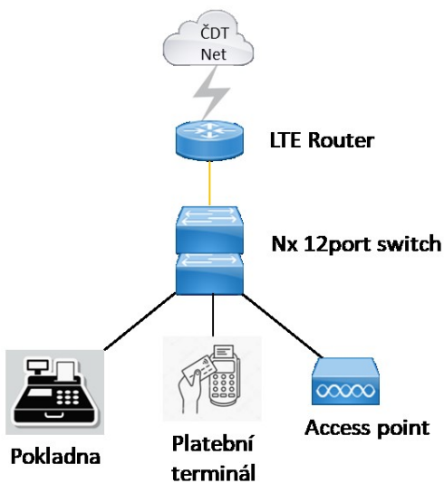
Obrázek 2 Ilustrační obrázek navržené komunikační infrastruktury dle Standardů ČD na lokalitách typu OBYČEJNÝ s LTE funkcionalitou (POKLADNA)
