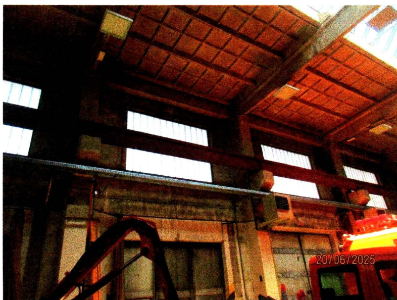
Foto č.5 U vyšších vrat je překlád rovněž tvořen keramickým panelem. Spodní část byla odříznuta, odbourána. Mělo by to jít i u ostatních vrat. Soudržnost keramických panelů opláštění je veliká. Odříznuté nadpraží se začistí zednickým způsobem - omítnutím.
