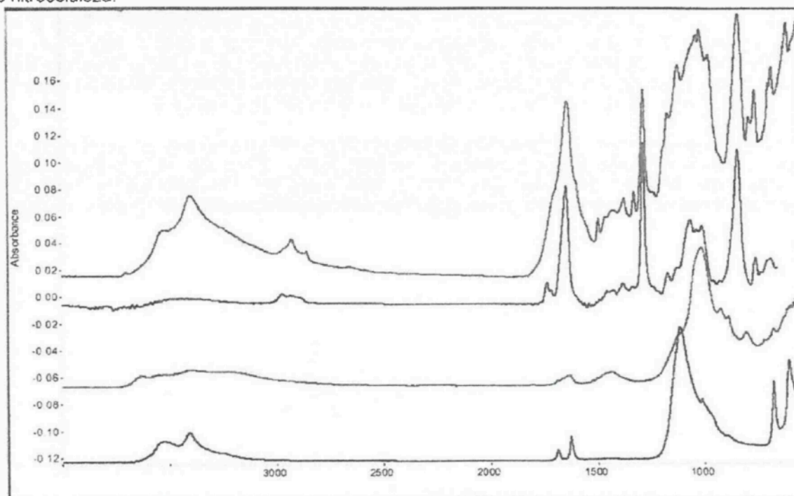
Obr.6: FTIR spektrum základní vrstvy laku z letadla Š16 spolu se spektry standardů.. Pojivém nátěru je nitrocelulóza.
