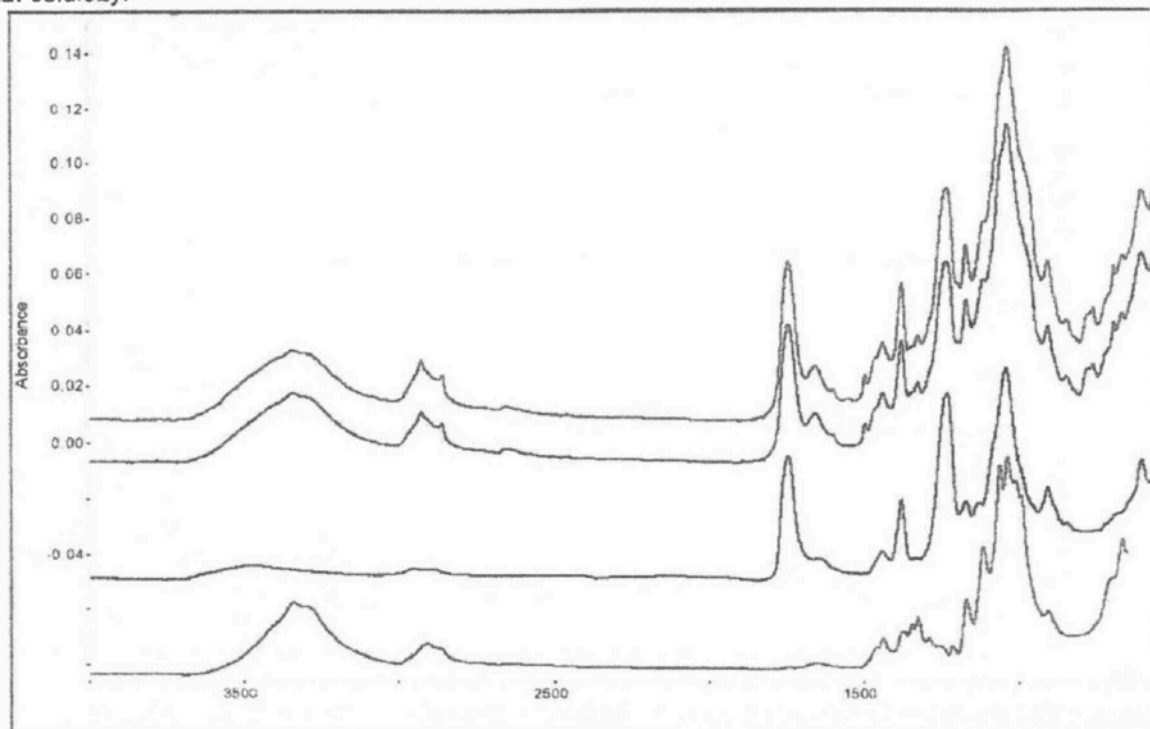
Obr.6: FTIR spektrum rubové základní vrstvy laku z letadla Š16 spolu se spektry standardů. Pojivém nátěru je acetát celulózy.
