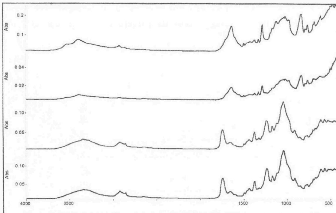
Obr.6: FTIR spektra všech změřených vzorků z letadla Š16. Jasně se liší licová spektra a spektra rubových
