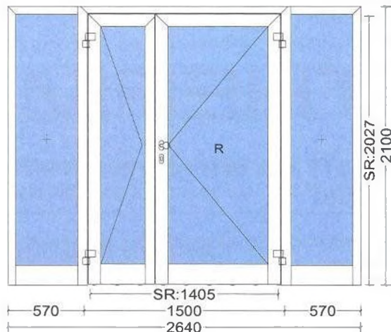
Pohled zvenku Systém: Heroal W/D 50 C SRM 3 Zaskl. lišta: Standard F 2
