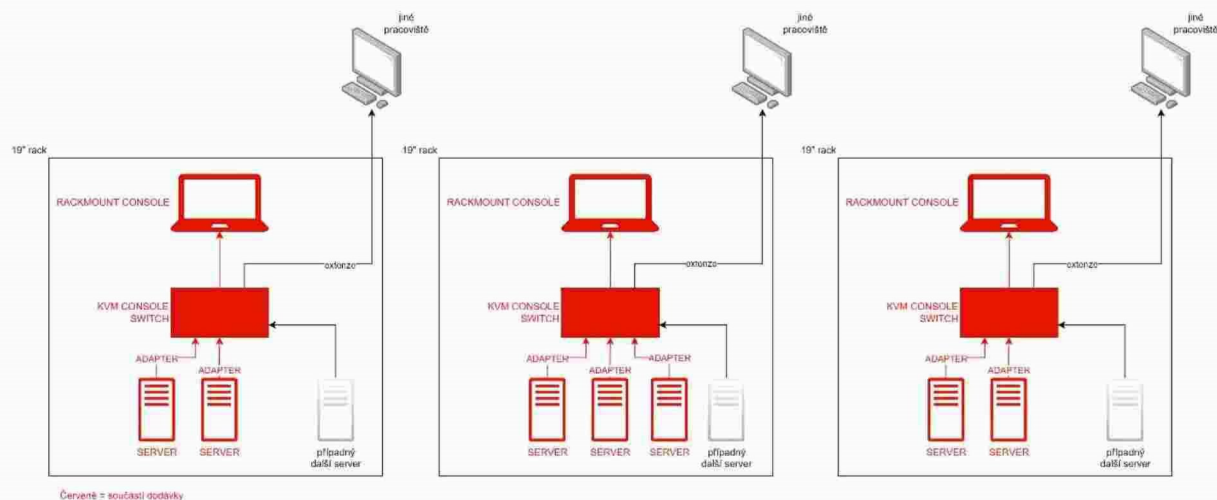
Obr. 1: Zjednodušené schéma zapojení hardwaru z dodávky.
