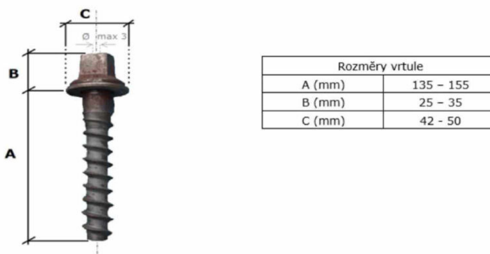
Obrázek 31 Vrtule
