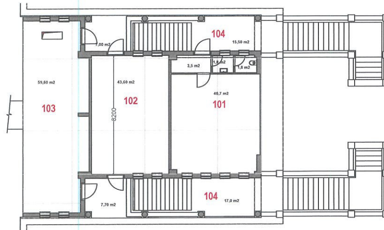
1 SUTERÉN -3,000
