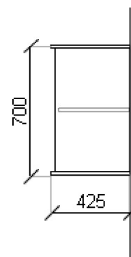
POHLED BOČNÍ
