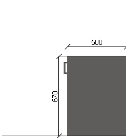
POHLED BOČNÍ
