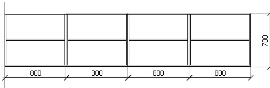
POHLED ČELNÍ
