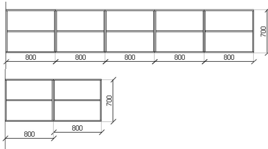
POHLED ČELNÍ
