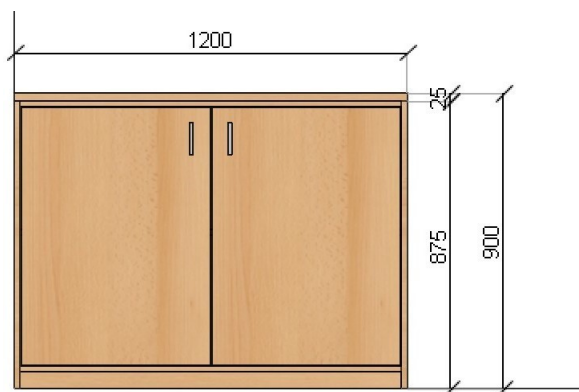
POHLED ČELNÍ
