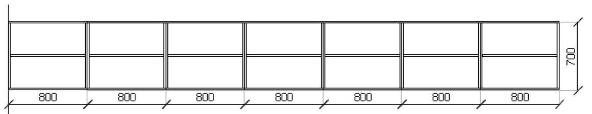
POHLED ČELNÍ
