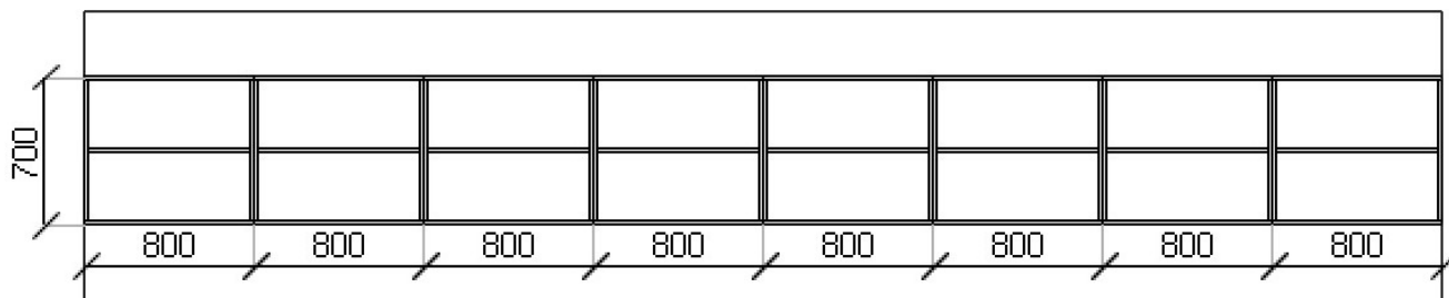
PŮDORYS
