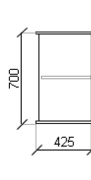
POHLED BOČNÍ
