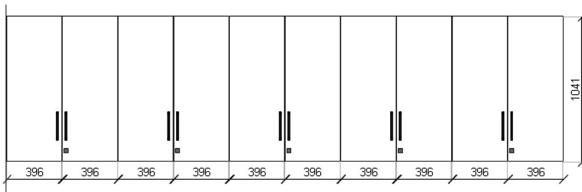
POHLED ČELNÍ
