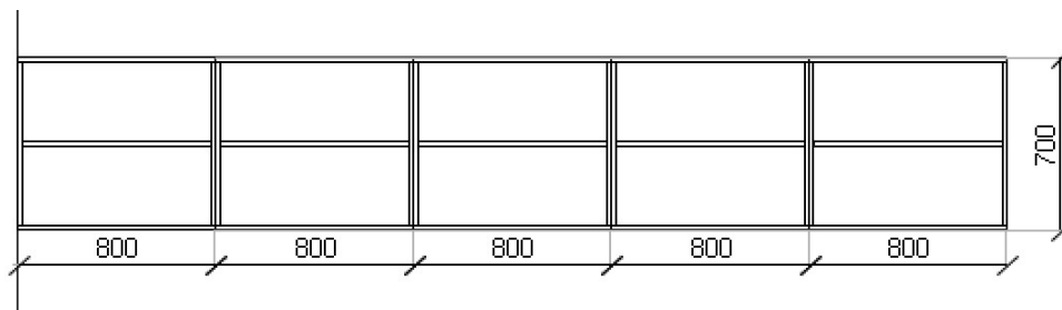
PŮDORYS
