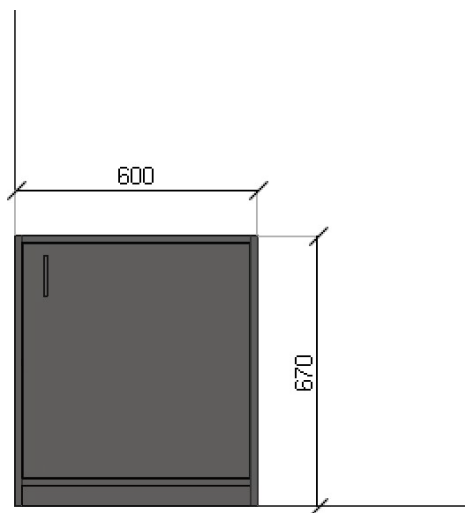
POHLED ČELNÍ
