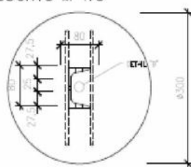
PŮDORYS M 1:5
