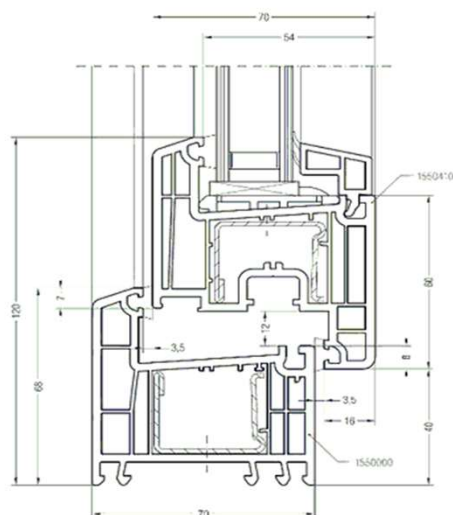
Detaily profilů
