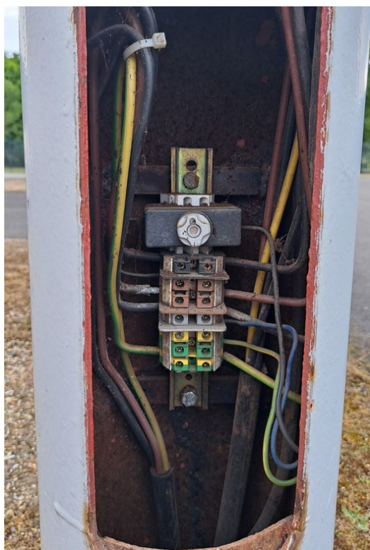
Obr. Č. 4 : stožárové svorkovnice
