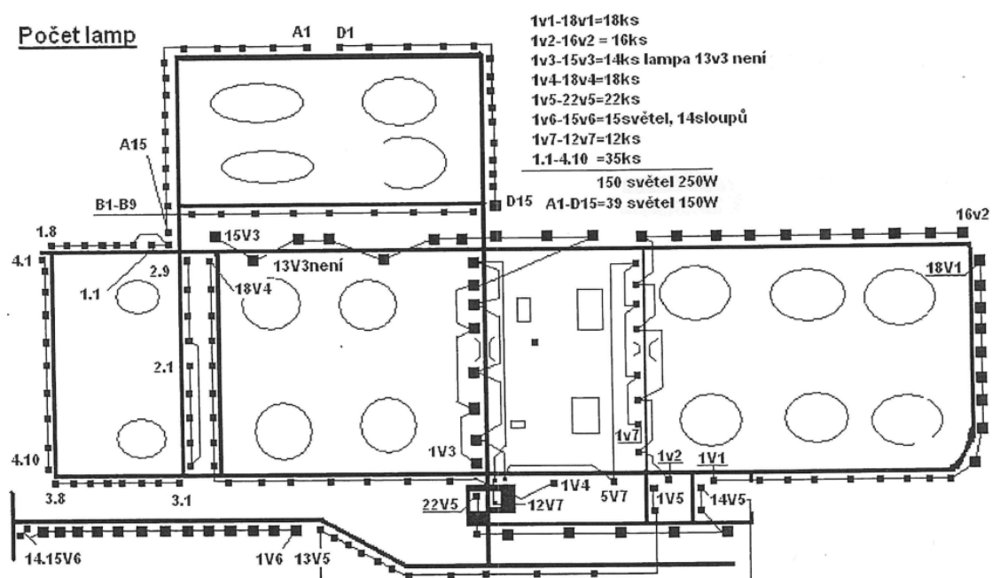
Obr. 2: Rozmístění stožárů
