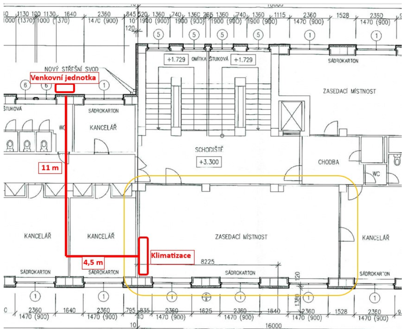
Nákres č. 3 klimatizace
