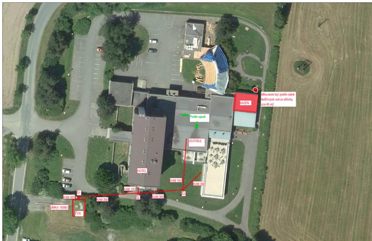
Obrázek 1: Náčrt vedení splaškové kanalizace z hotelu a umístění ČOV
