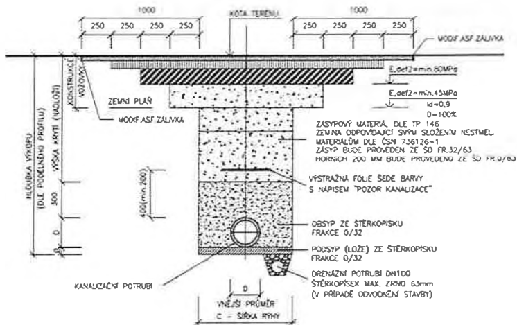
Konstrukce vozovky dle TP 170 D1-N-6-V-PIII
