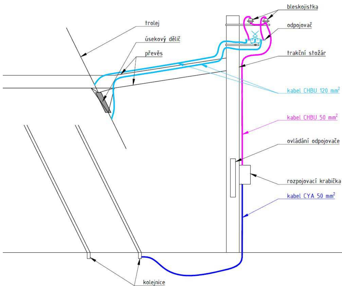
Obr. 33: Zapojení úsekového dělení
