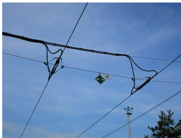
Obr. 41: Umístění návěstidla úsekového dělení
