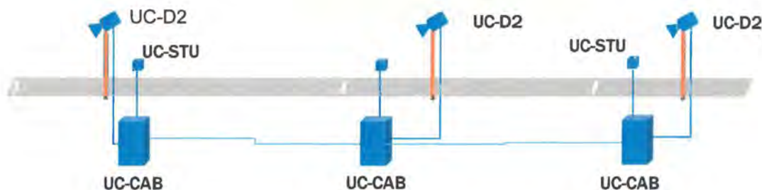
Obr.19: Kaskádová varianta
