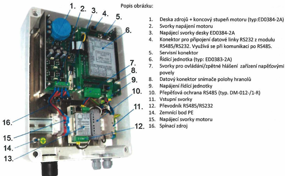
Obr.1: Základní popis elektroniky
