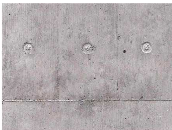
b) z pohledové strany u nosníkového nebo atypického bednění (vlevo bednění / vpravo povrch betonu)
