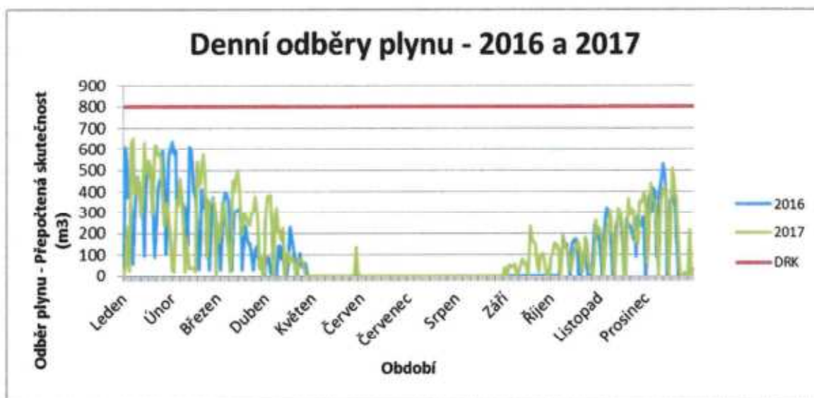
Ilustrační obr.5 – srovnání denních spotřeb ZP
