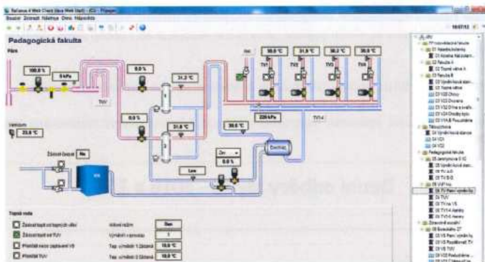
Ilustrační obr.2 - Monitoring výměňkové stanice tepla
