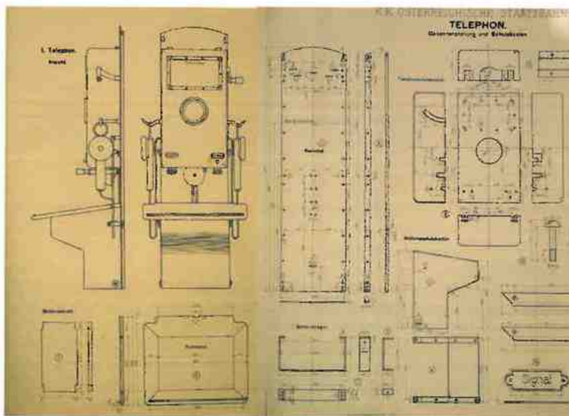
Výkres původního provedení přístroje
