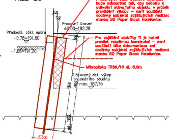
ŘEZ E3-0
