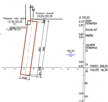
ŘEZ E3-0
