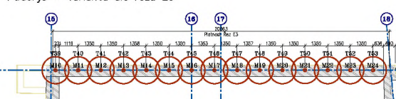
Pádorys – varianta dle řezu E3
