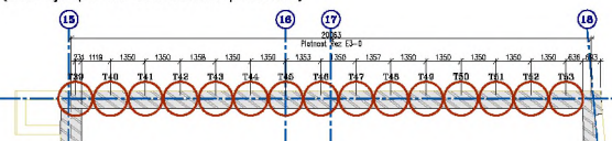
Pádorys – varianta dle řezu E3-0 (Bez výkopu na sousedním pozemku)
