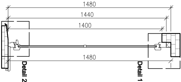
SVISLÝ ŘEZ B-B
