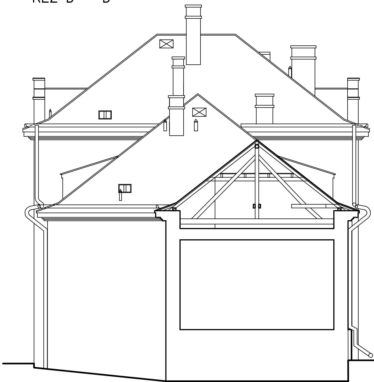
ŘEZ D – D
