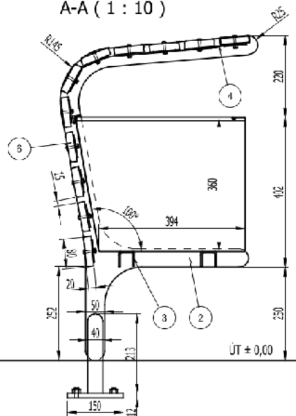
A-A (1 : 10)
