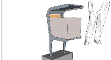
Do připraveného betonového základu se vyvrtají otvory a na chemickou kotvu osadí závitové tyče, které zajistí upevnění koše na místě.
