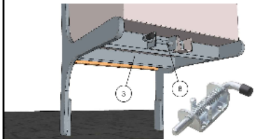
Dále je nádoba zajištěna pružinovou západkou a okem navazným na dně nádoby.
