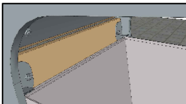
Odpadní nádoba je uchycena na místě samotnou konstrukcí koše, jako západky profi pohybu slouží úhelníky v horní části konstrukce.
