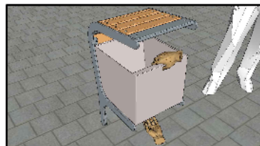
Demonstrace odejmutí nádoby: Jednou rukou posuneme kolík pružinové západky. Druhou rukou tahem nahoru za pomoci úchytu odejmeme nádobu.
