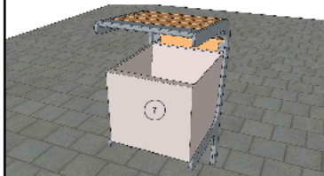
Koš je vybaven odnímatelnou odpadní nádobou z nerezového plechu o objemu 48 litrů.
