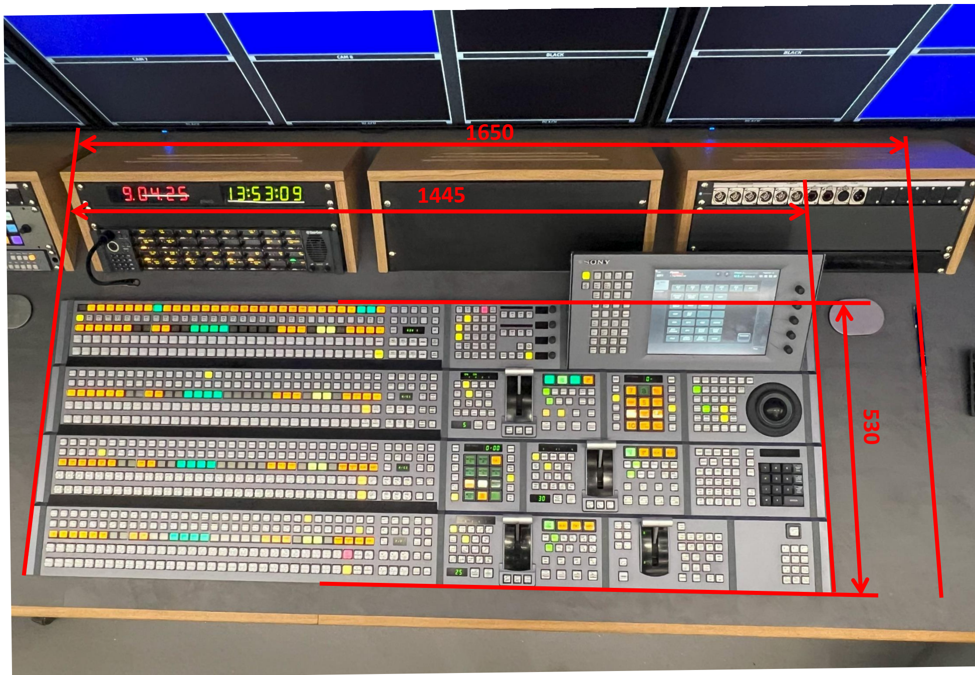
Obr. 2 – Rozměry stávajícího ovládacího panelu, možnost rozšíření otvoru při demontáži zásuvky 230 V
