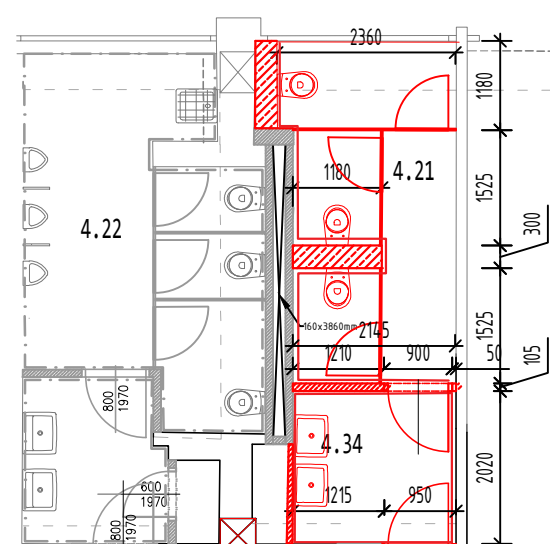
Nové konstrukce M 1:100
