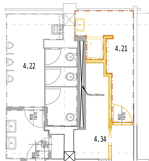
Bourané konstrukce M 1:100
