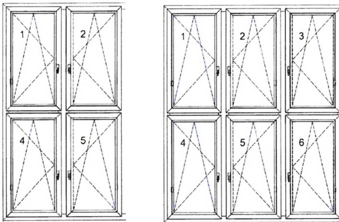
Obr. 3 - Rozčlenění oken
