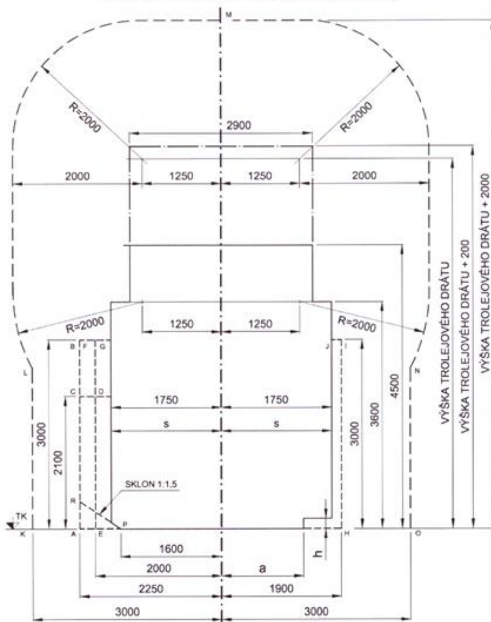
Obrázek 6 – průjezdny průřez pro jednokolejně trati
