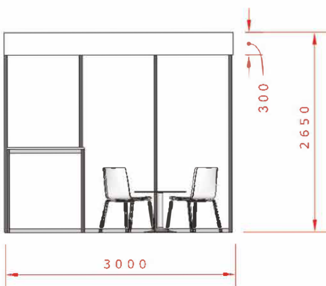
pohled čelní M 1:50
