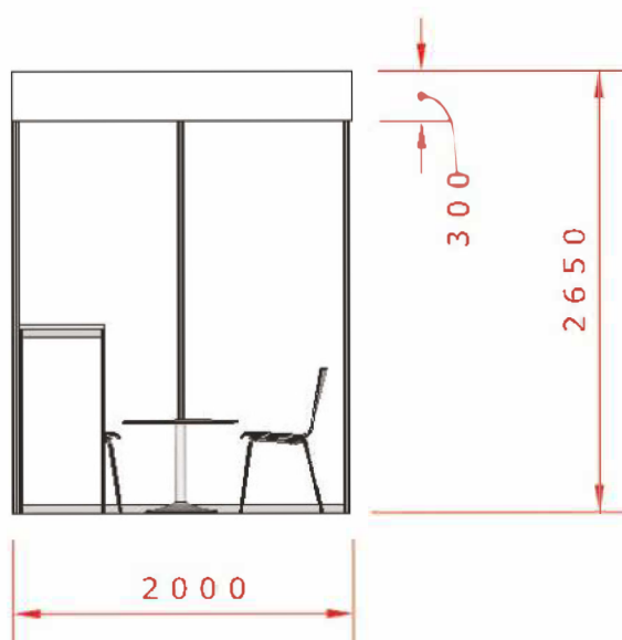
pohled čelní M 1:50
