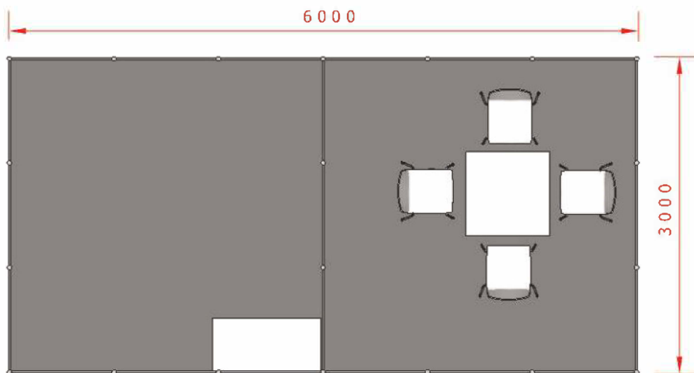
půdorys M 1:50
