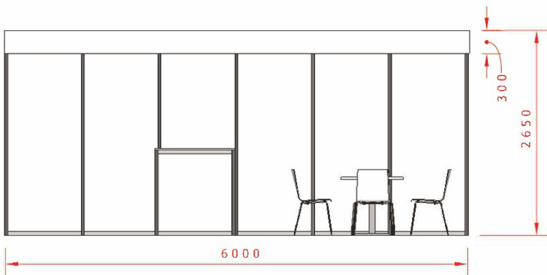
pohled čelní M 1:50
