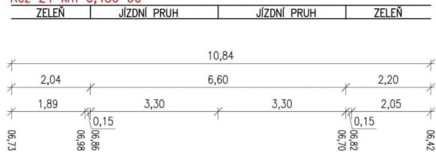
Řez 24 km 0,480 00
