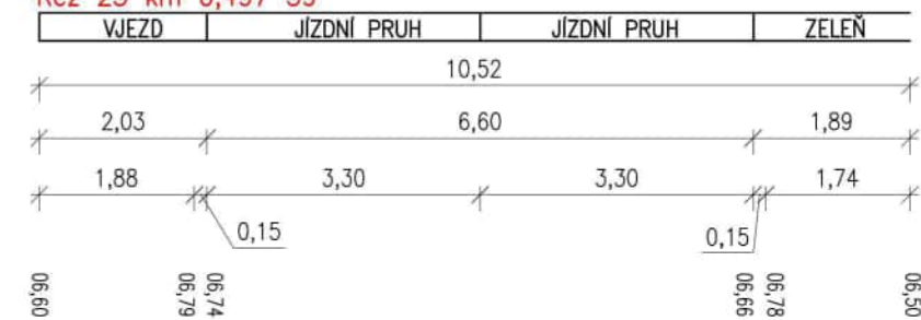
Řez 25 km 0,497 39
