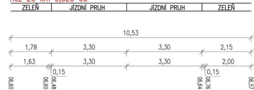
Řez 26 km 0,523 00
