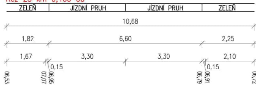
Řez 23 km 0,460 00
