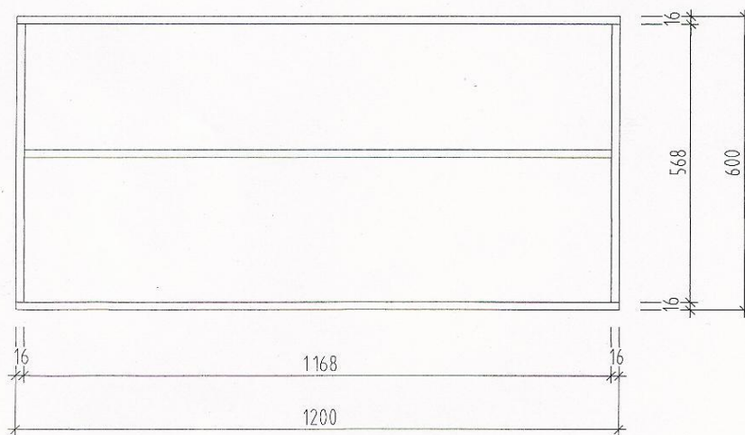
ČELNÍ POHLED
