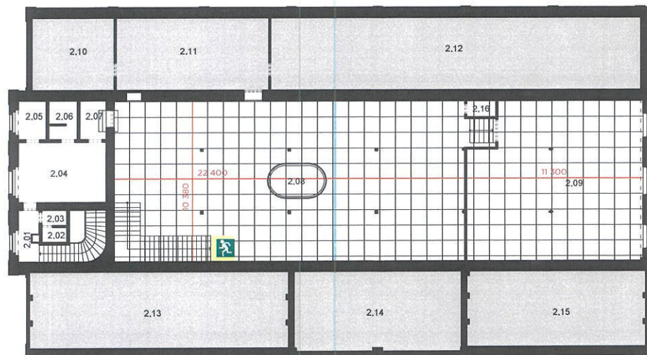
SCHEMATICKÝ PŮDORYS 2.NP
