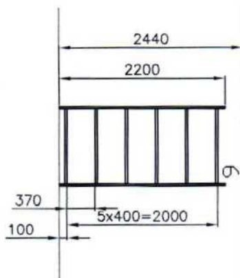
POHLED NA SLOUPEC :
