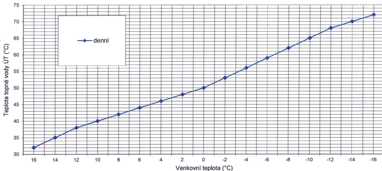
Teplotní křivka
