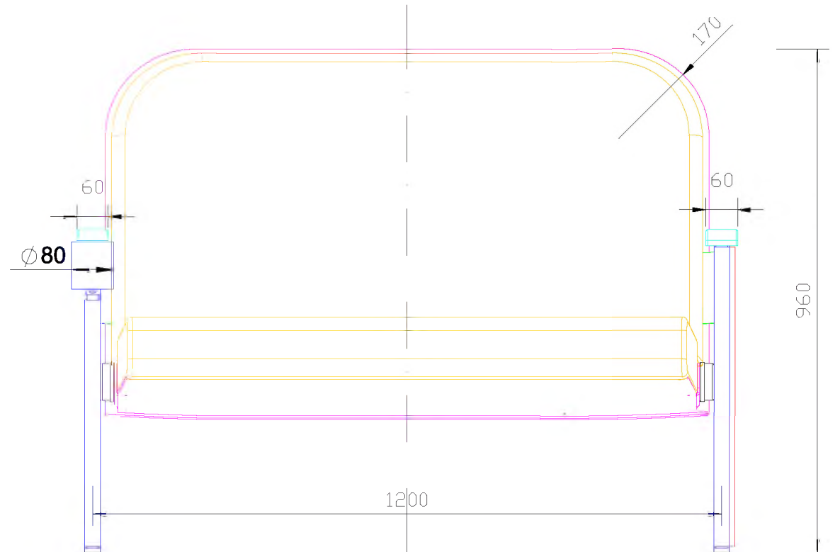
ČELNÍ POHLED
