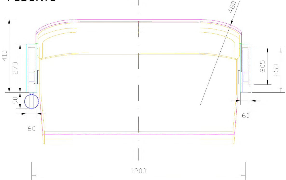
ČELNÍ POHLED
