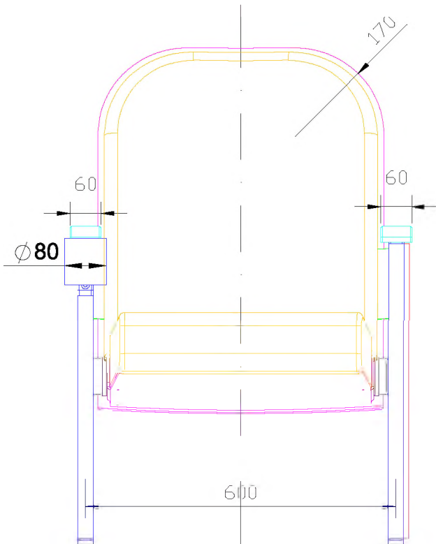
ČELNÍ POHLED
