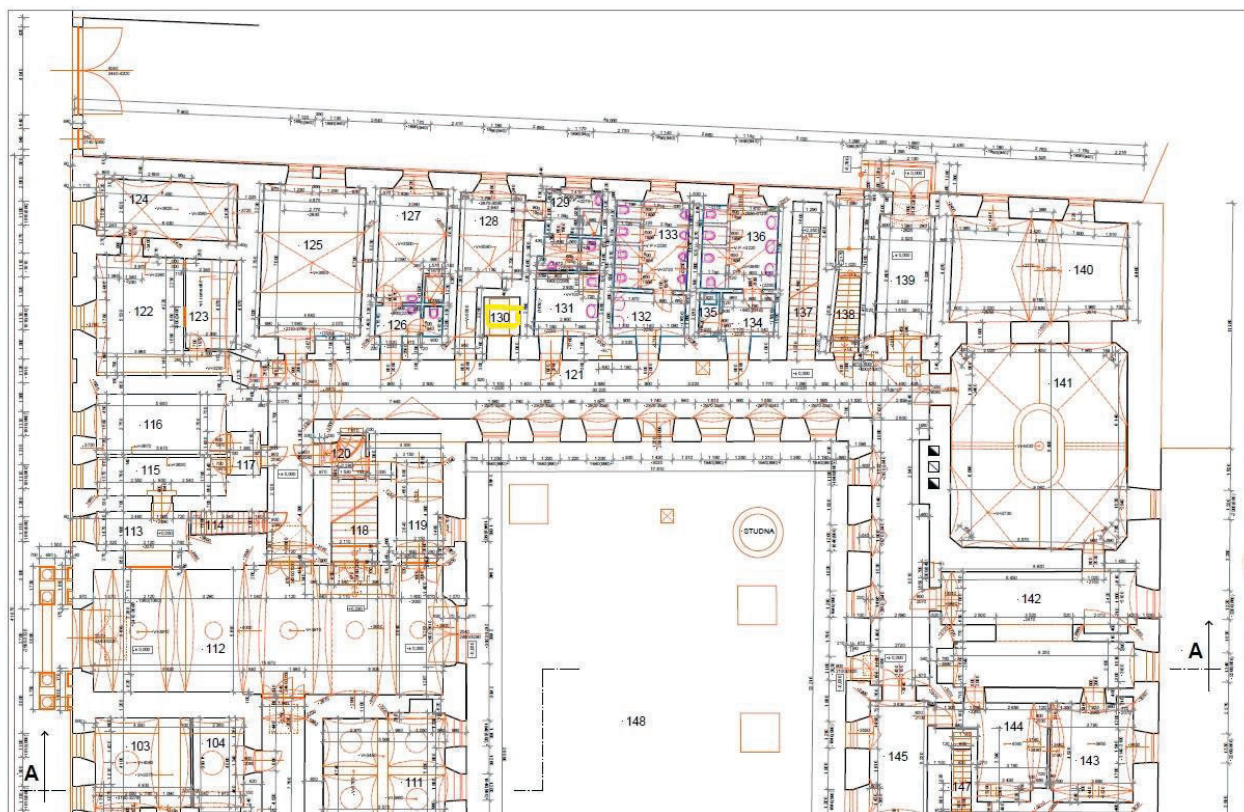
Obrázek 2: Umístění osobního výtahu v budově (výřez, 1. NP, místnost č. 130)
